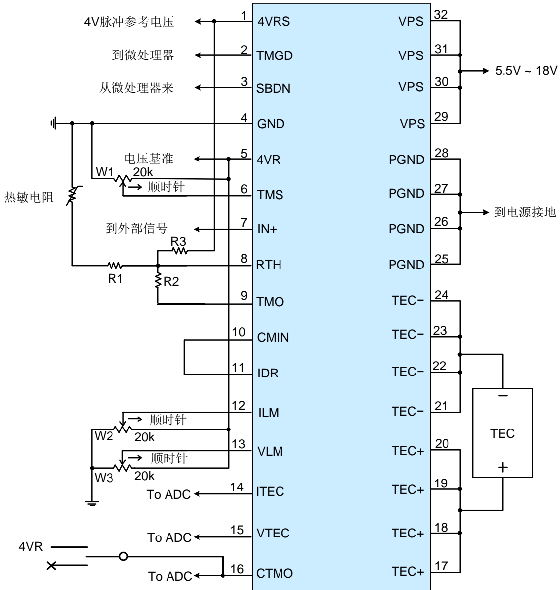
图 8.2. TEC18V10ADAPID 和 TEC18V10ASAPID 的连接
