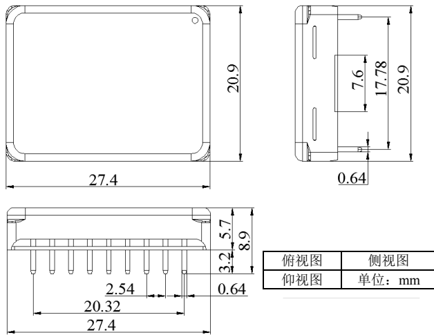
图 11、DIP 封装驱动器的尺寸
