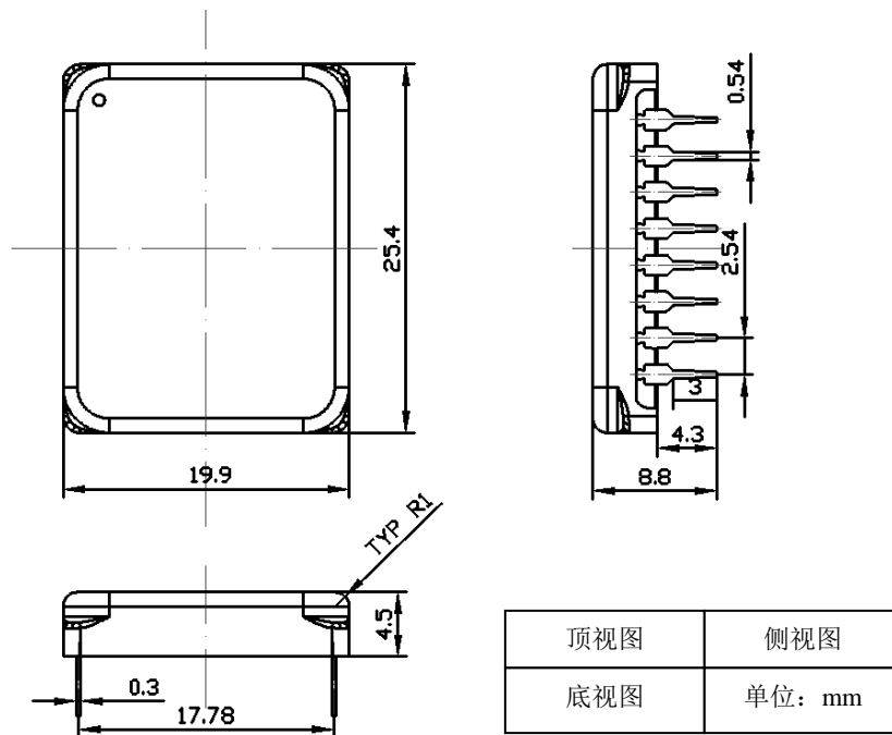
图15、TEC5V6A-D的DIP封装尺寸图
