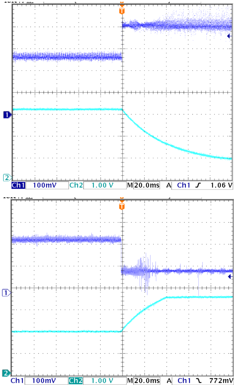
图 13、 V_{TEC} 与 V_{TMO} 波形图
