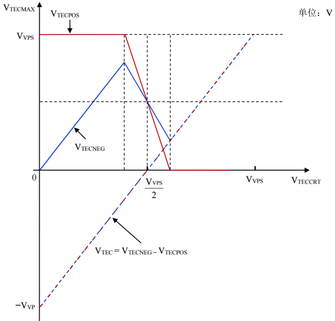
图 5、 V_{TEC_{MAX}} & V_{TEC_{CRT}}
