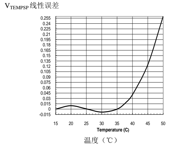
图 12、 V_{TEMPSP} 与温度的线性误差
