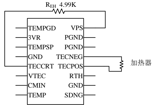
图 6.2、驱动一个加热器 < 3.3V @ <= 3A
