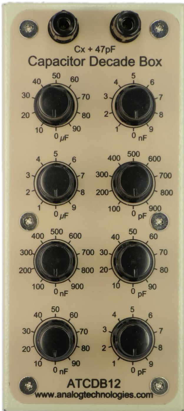
图 2、ATCDB12 俯视图
