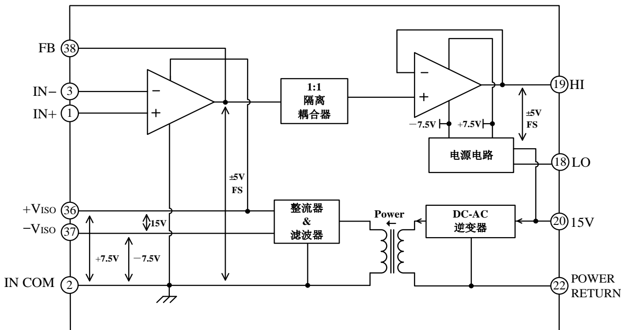
Figure 2. AD202KNATI 的功能方框图
