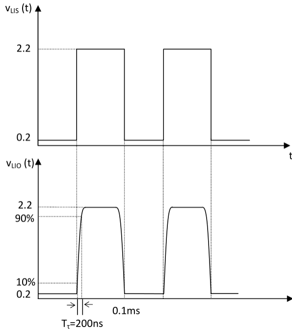
图 14、大信号调制
