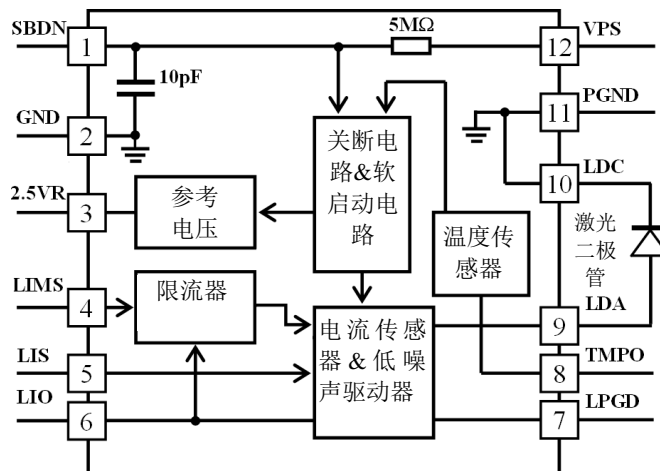
图 4、方框图
